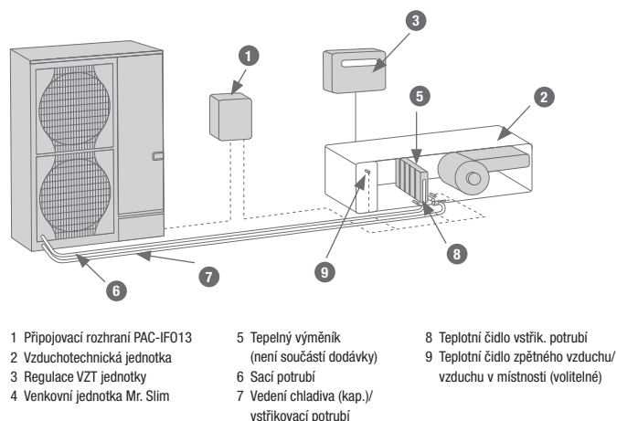
Použití připojovacího rozhraní s větracím systémem
